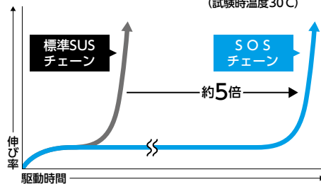
駆動時間による伸び率の比較 (試験時温度30℃)
