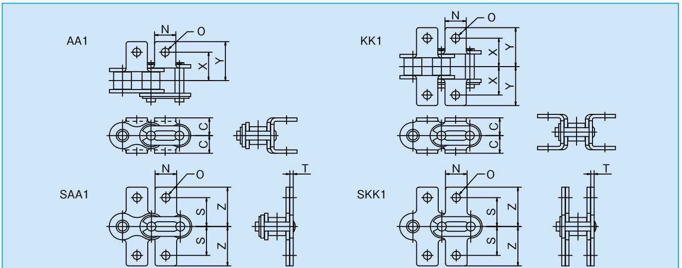
○寸法表
