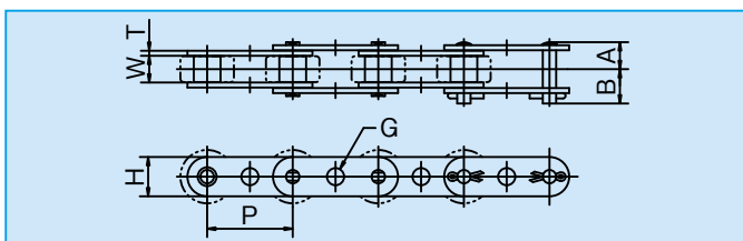
○寸法表
